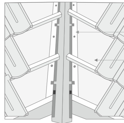
Contrașipcă 30x50 mm Folie anticondens
